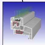
Onderdorpel in NL Plus profiel
